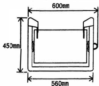
☆ ベルトコンベア前面図 (各タイプ共通)
