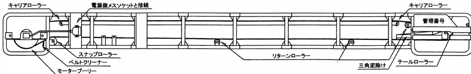
☆ ベルトコンベア前面図 (各タイプ共通)
